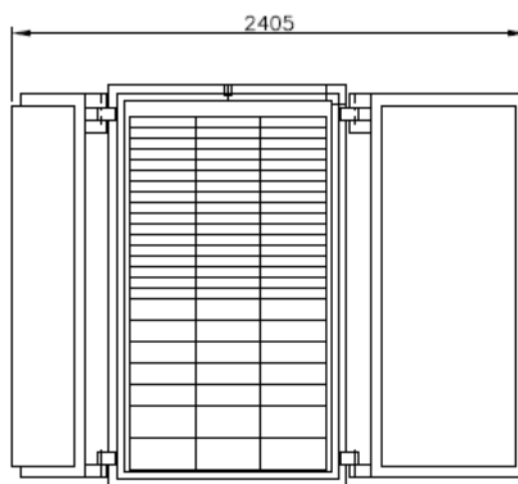
Mod. 1902 con 2 porte – 3 blocchi LSH
