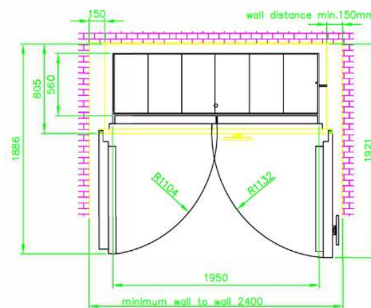
Mod. 1904-6 DS 55 per 6 colonne LSF accessibili con porte a 90°- ingombri
